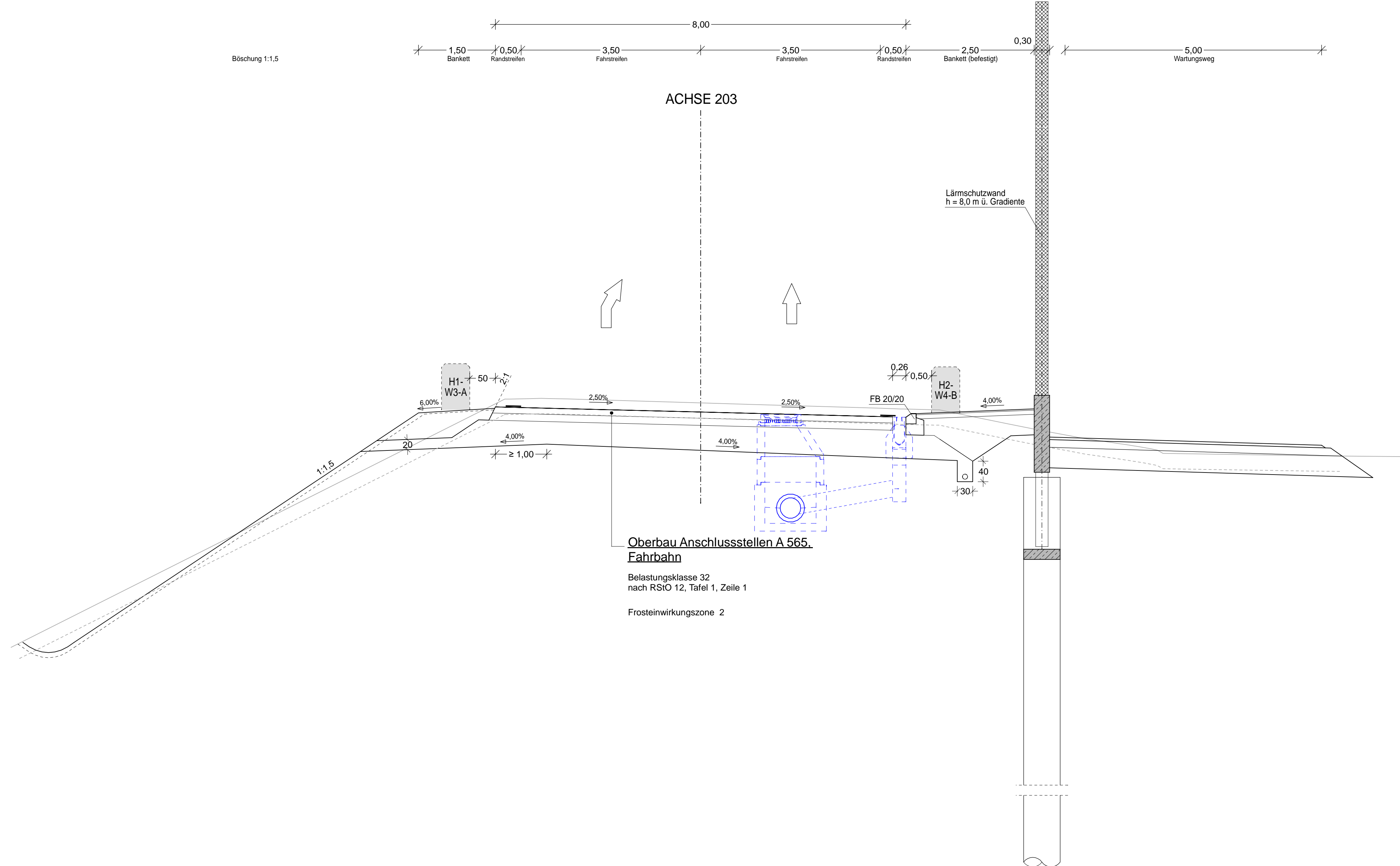
Querschnitt Einfahrt Edenich, km 0+050,000, M.: 1:50
