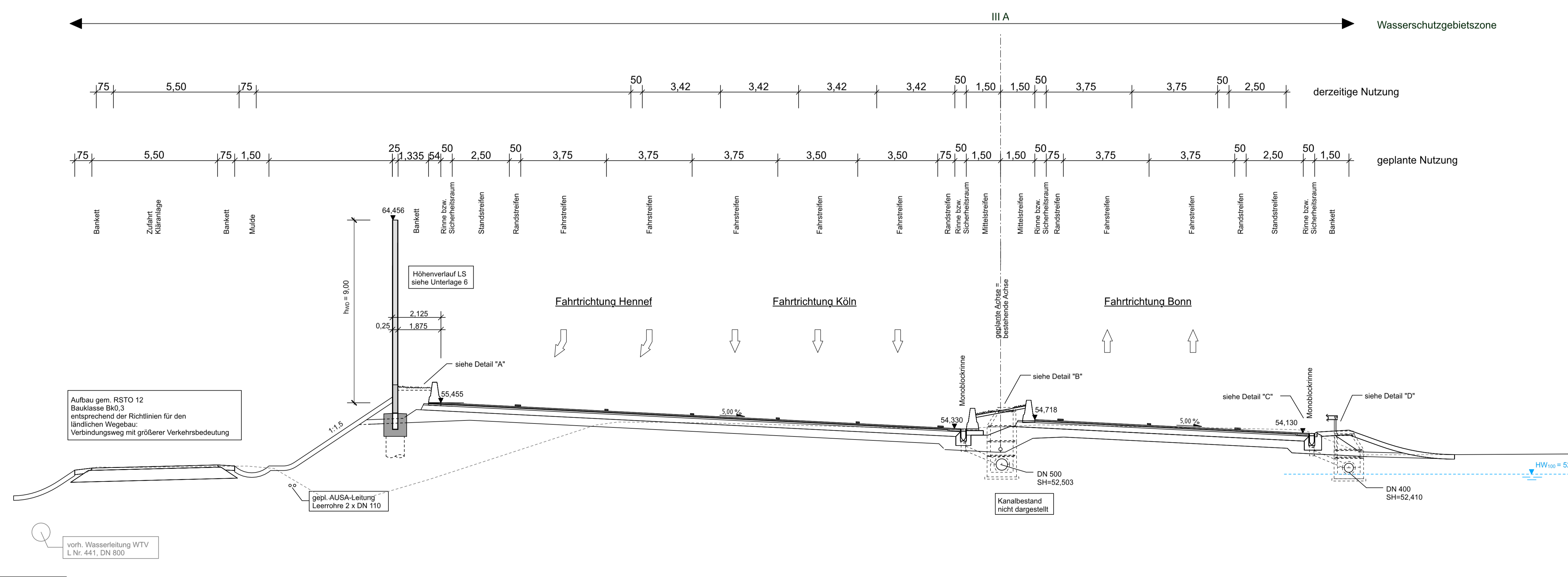
Querschnitt Maßstab 1:100 23+700.000
