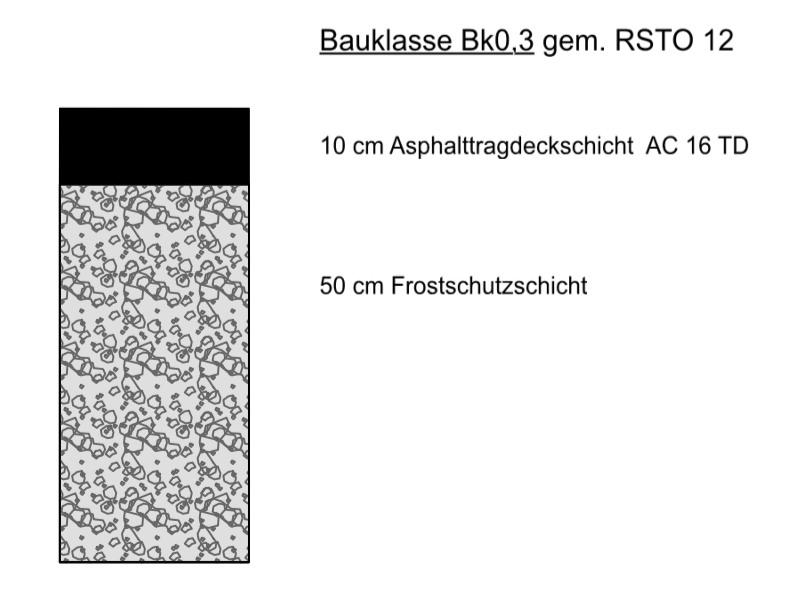
Deckenaufbau Zufahrt ZABA / Kläranlage Maßstab 1:10
